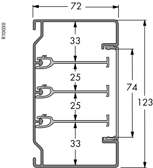
TEK-123/72 Til montering på væg eller på konsoller.
