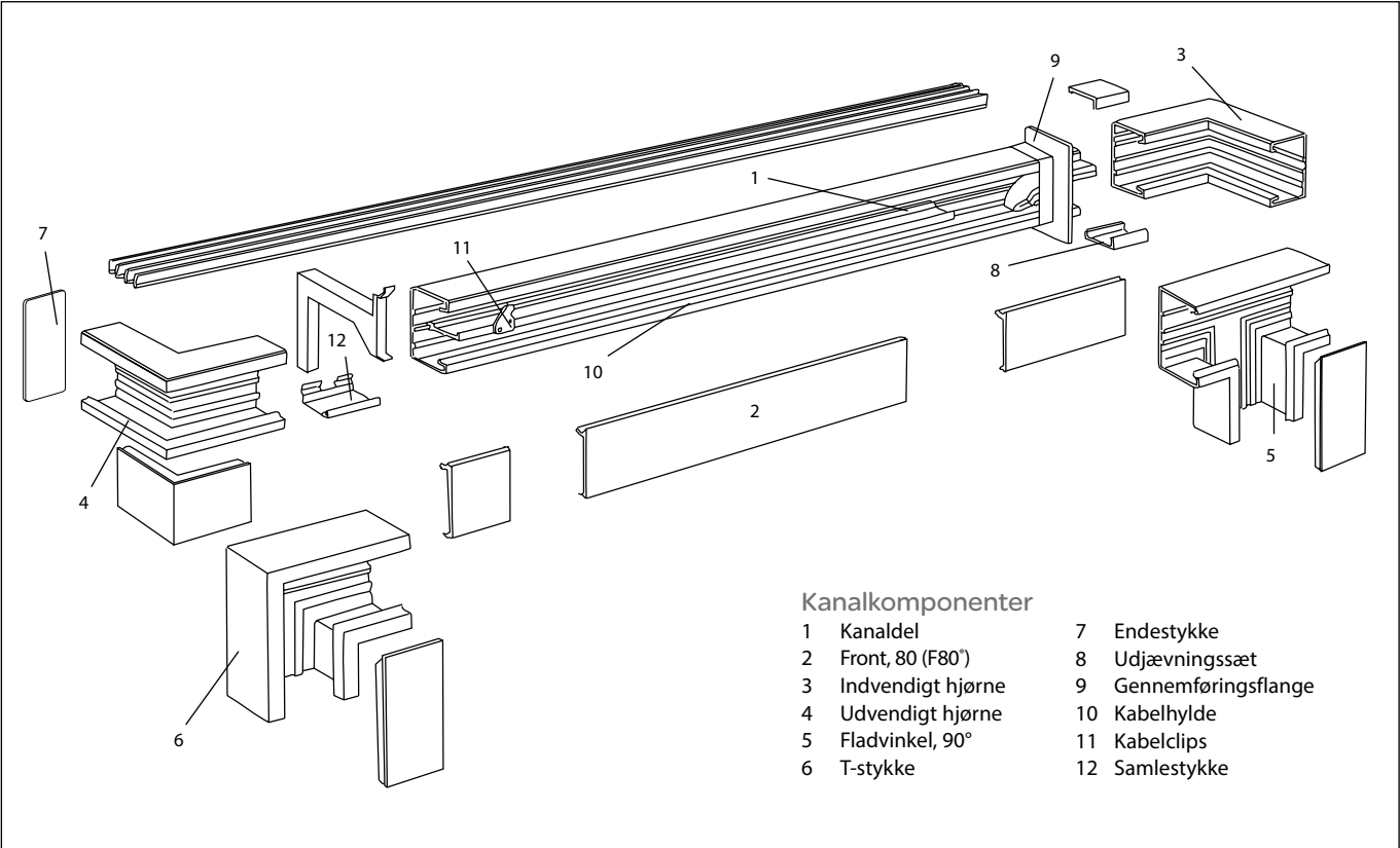
TEK-100/52 Til montering på væg eller på monteringsbrikker.
