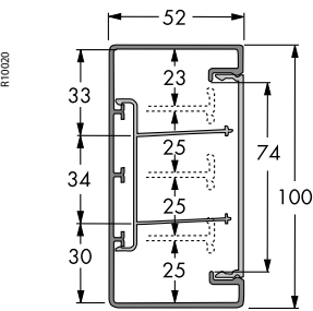
TEK-100/52 Til montering på væg eller på monteringsbrikker.
