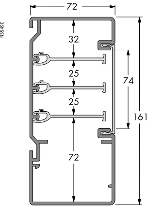
TEK-161-3/72 Til montering på væg eller på konsoller.
